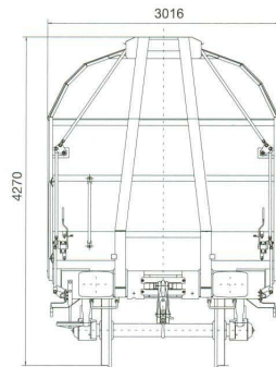
ČELNÝ POHĽAD
